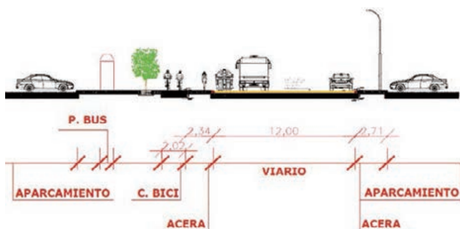
Plano del alzado de calle, en una de las actuaciones previstas en el barrio.
