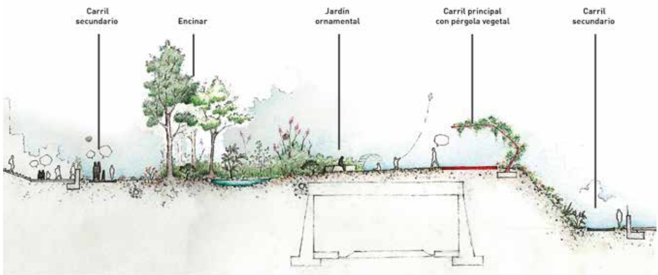
Sección transversal del proyecto de cubrimiento.
